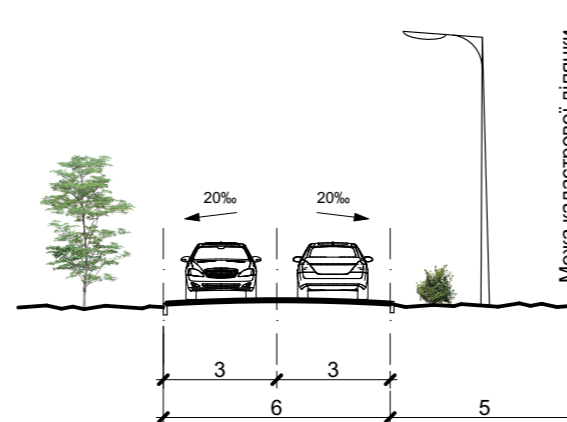
Переріз 4 - 4
