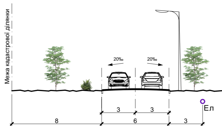
Переріз 1 - 1
