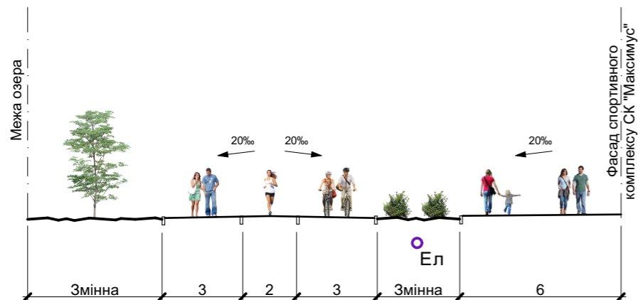
Переріз 3 - 3
