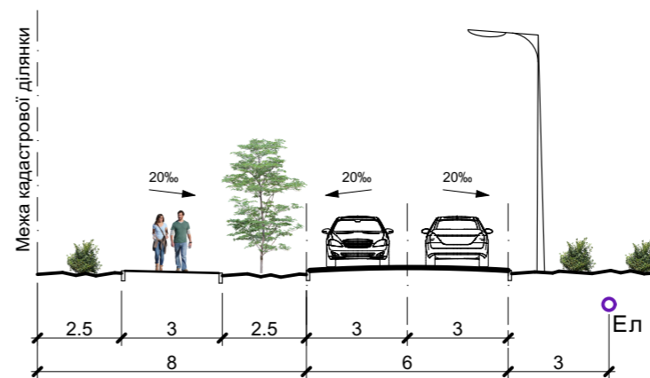
Переріз 2 - 2
