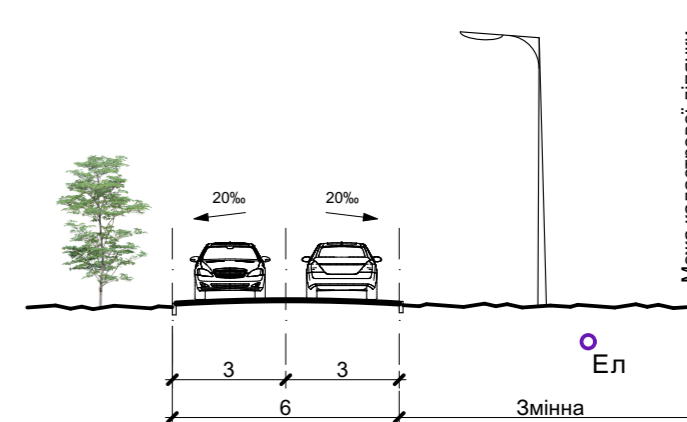
Переріз 5 - 5
